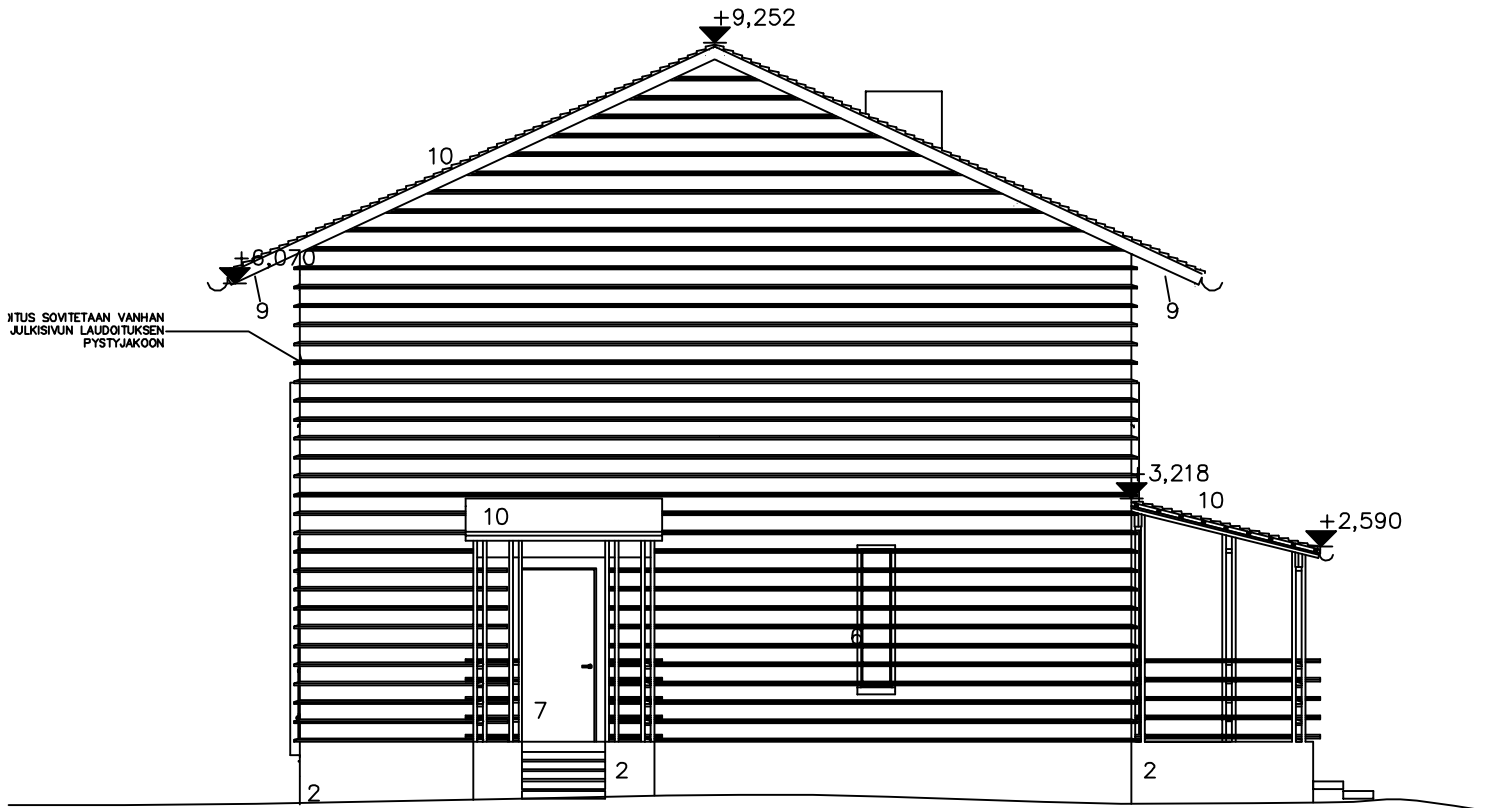
JULKISIVU LÄNTEEN 1:100
