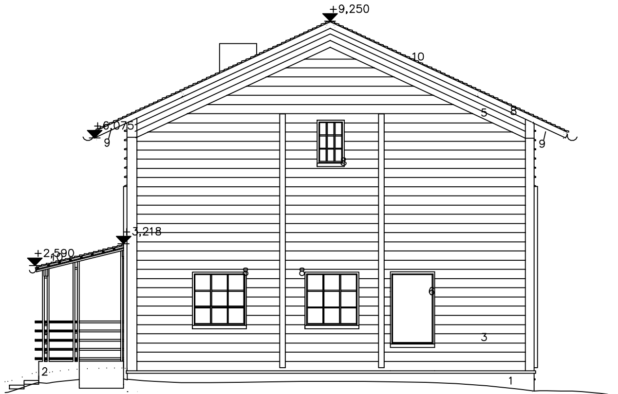
JULKISIVU LÄNTEEN 1:100
